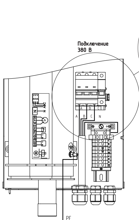
Рис.3 Схема подключения электроводонагревателя
